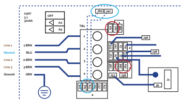
Ligne triphasée 380V III BP21G1WL
